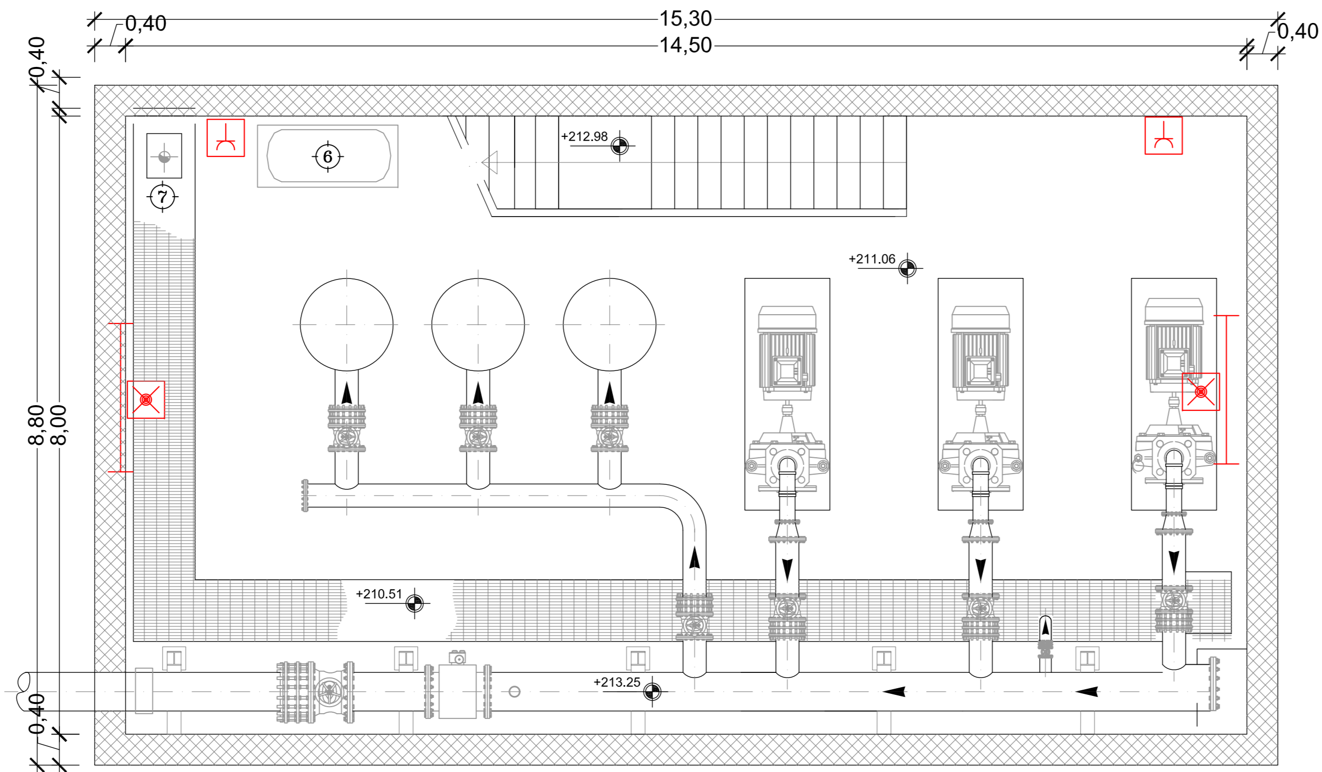
PIANTA A QUOTA +222.50
