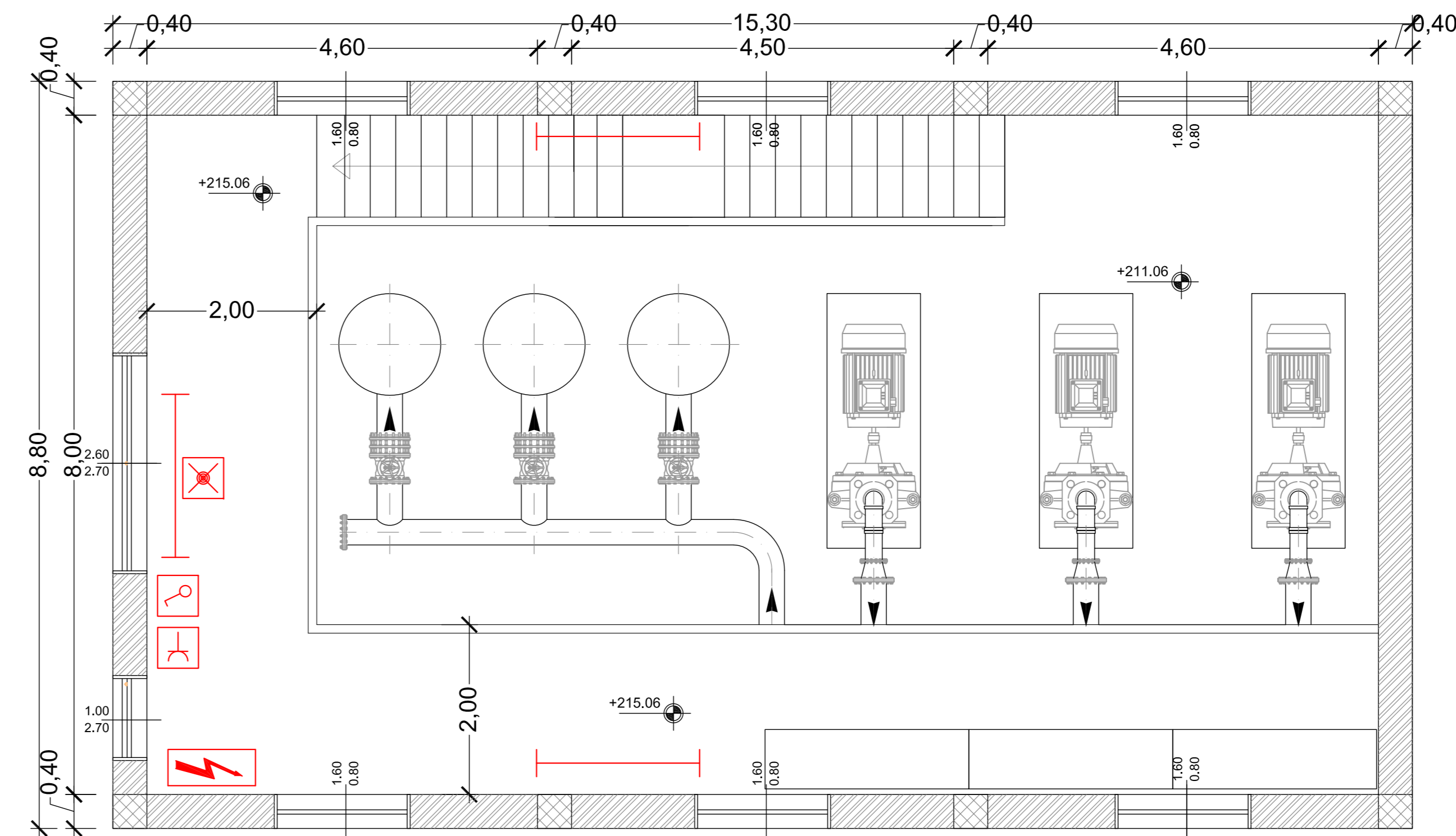
PIANTA A QUOTA +225.00
